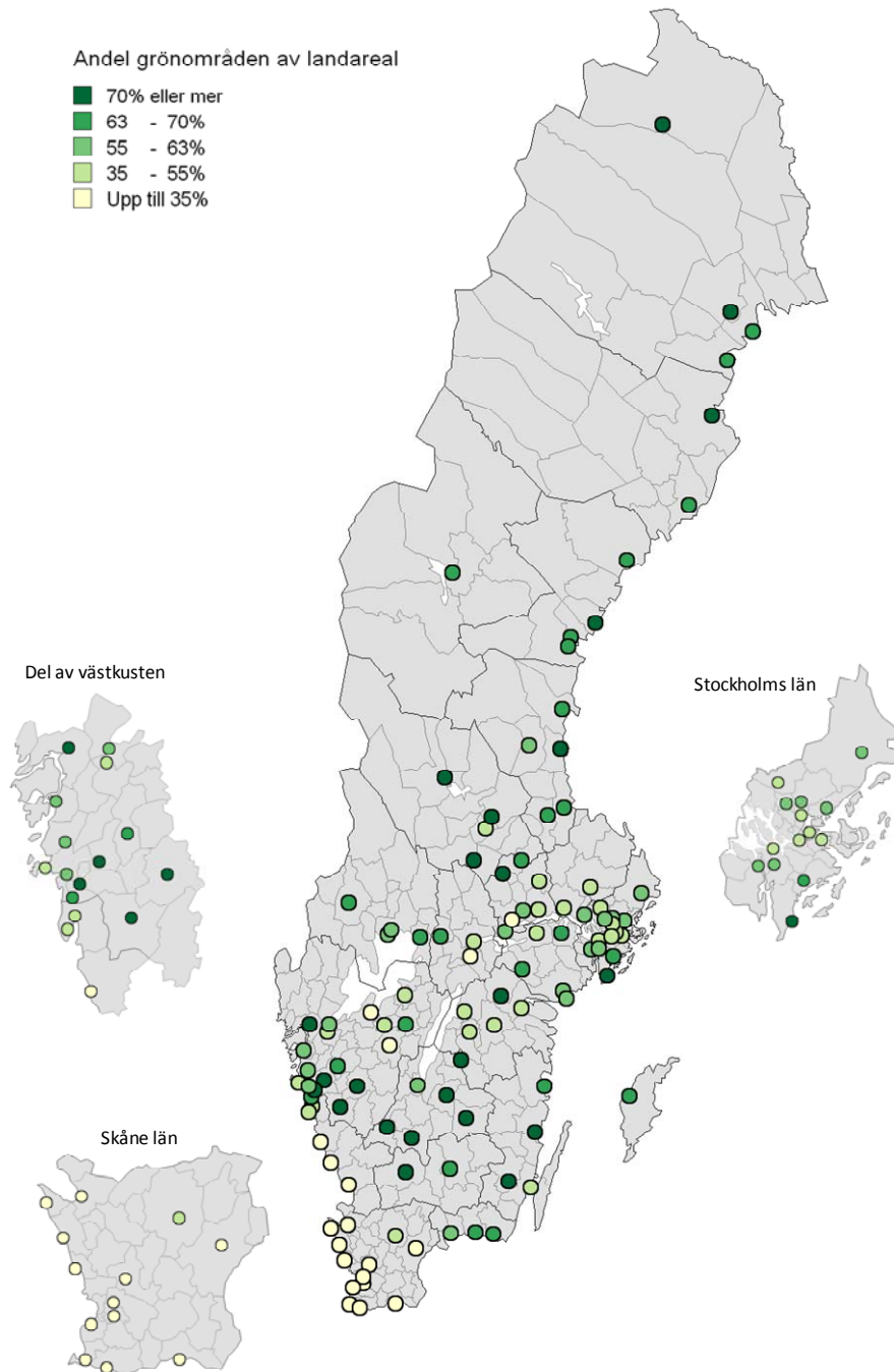
Karta 3. Andel grönområden inom tätort med omland om tre kilometer, procent av landareal. Tätorter med fler än 10 000 invånare, 2005
