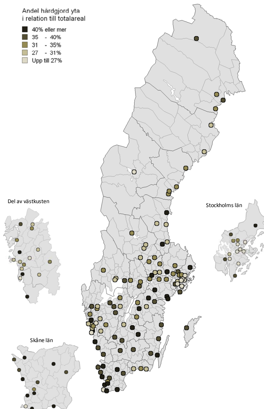
Karta 2. Andel hårdgjord yta inom tätort, procent av tätortsarealen. Tätorter med fler än 10 000 invånare, 2005
