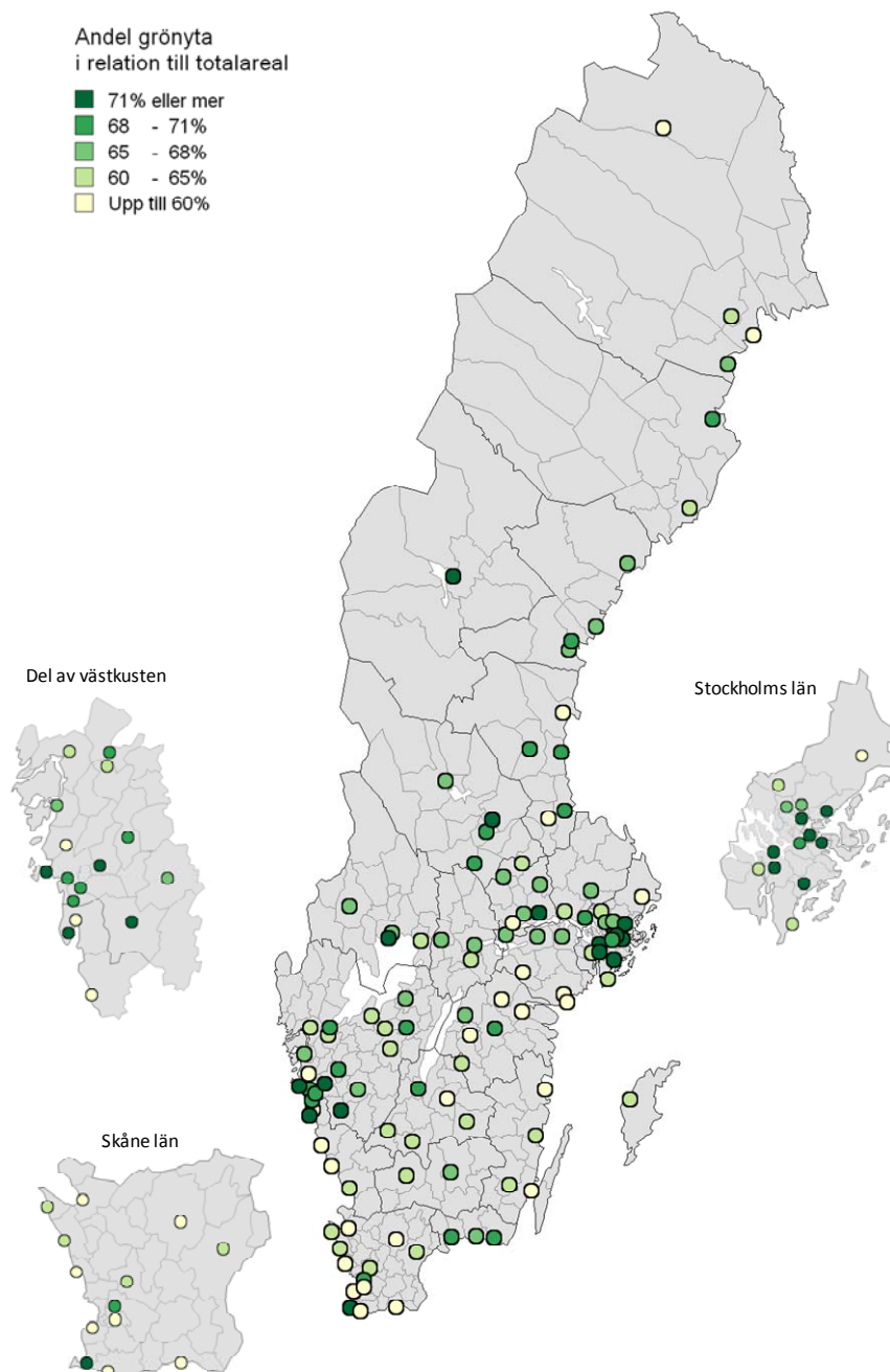
Karta 1. Andel grönyta inom tätort, procent av tätortsarealen. Tätorter med fler än 10 000 invånare, 2005
